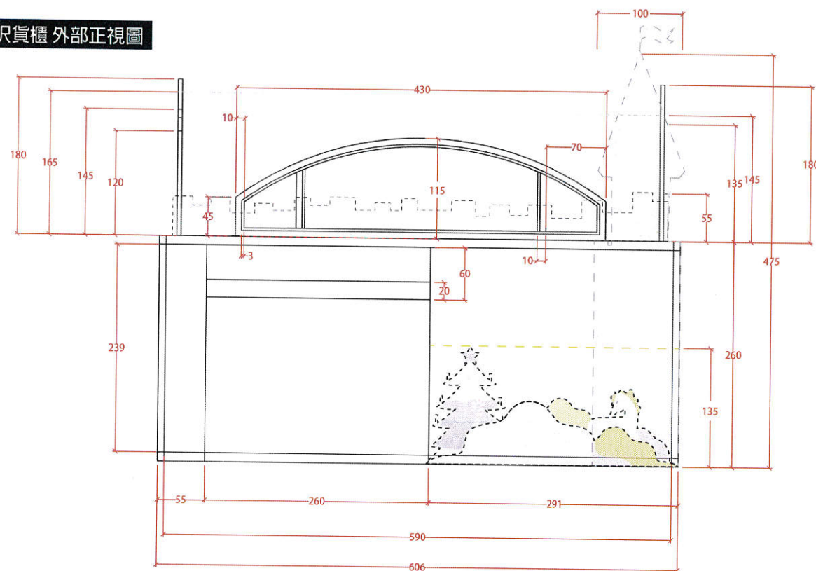
20呎貨櫃 內部正視圖
