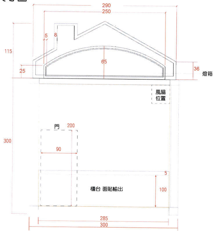
正立面
