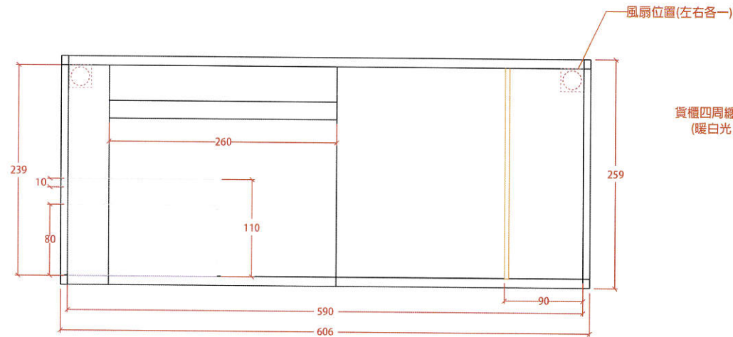
木頭20呎貨櫃 側視圖
