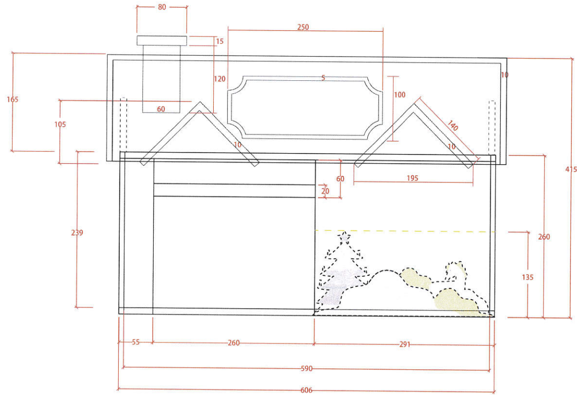
木頭20呎貨櫃 內部正視圖
